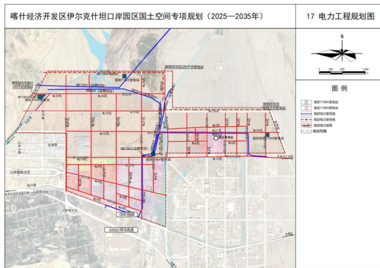
图2-3-12 伊尔克什坦口岸园区电力工程规划图
