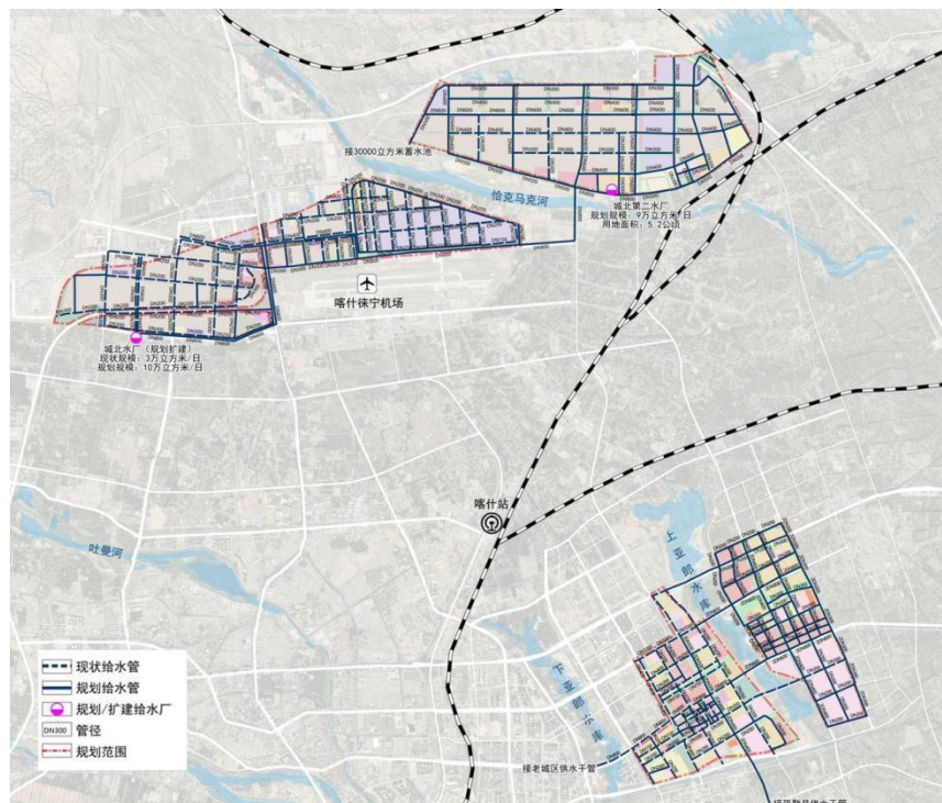
图2-3-6 喀什经济开发区（主体园区）给水工程规划图
