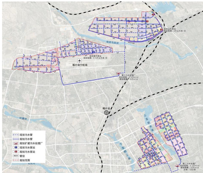
图 2-3-7 喀什经济开发区（主体园区）排水工程规划图
