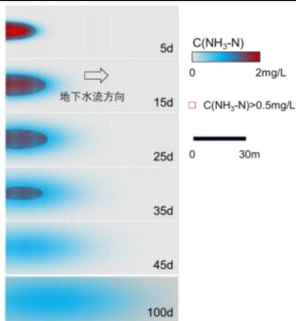
图5-3-3 \text{NH}_3\text{-N} 的污染羽在地下水中的分布情况
