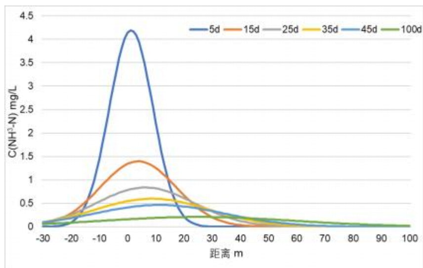
图5-3-4 \text{NH}_3\text{-N} 浓度分布情况
