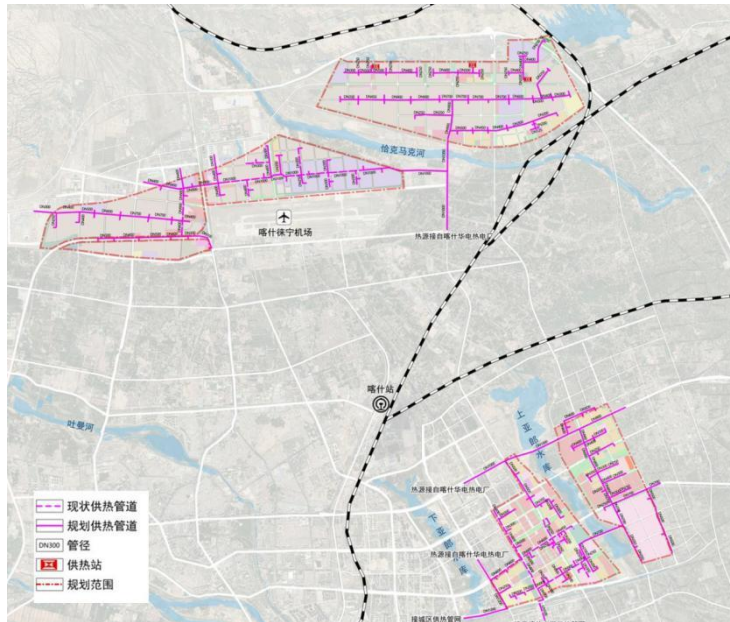
图2-3-16 喀什经济开发区（主体园区）供热工程规划图
