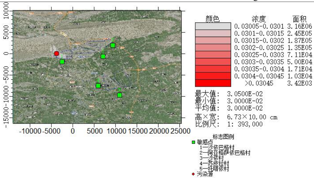
图5-2-11 NO 2 日均落地浓度叠加值网格图 (mg/m 3 )
