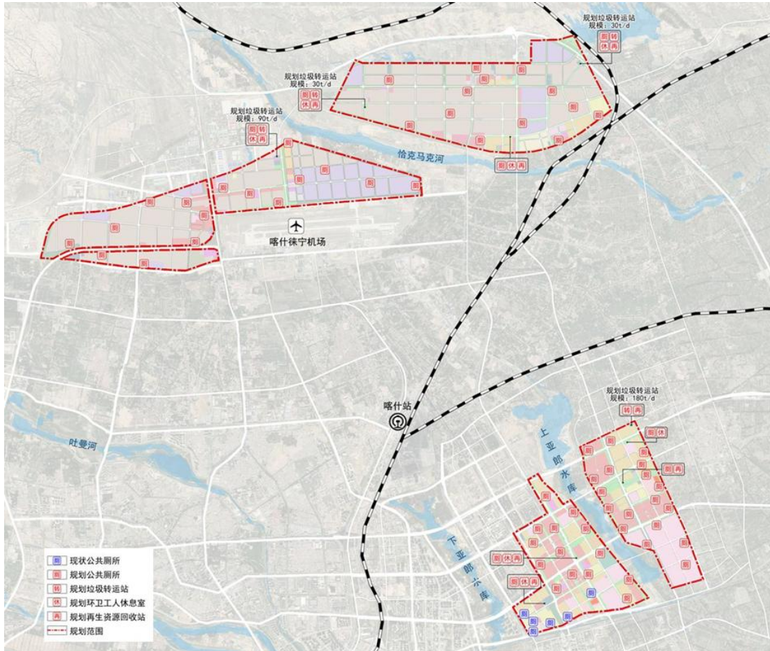
图2-3-18 喀什经济开发区（主体园区）环卫设施工程规划图
