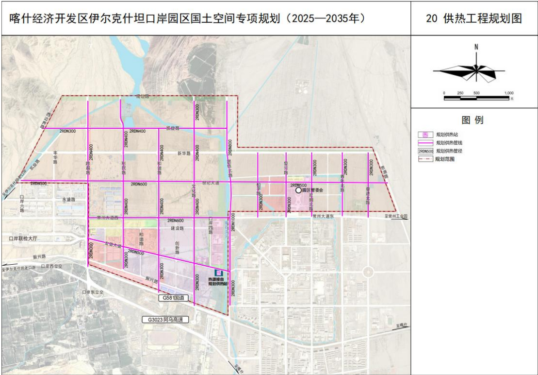
图2-3-17 伊尔克什坦口岸园区供热工程规划图
