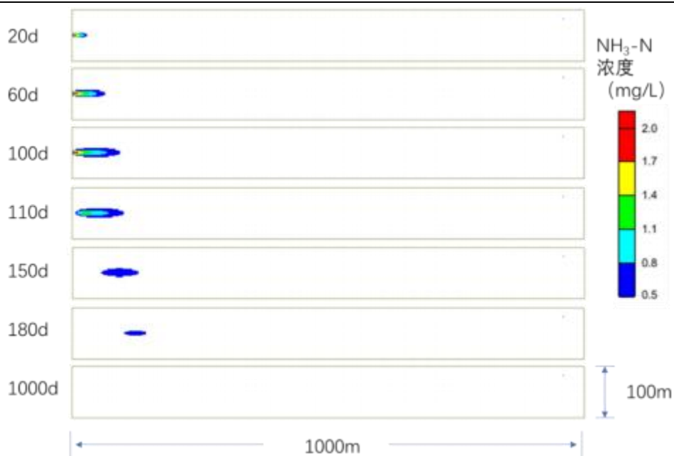
图 5-3-6 \text{NH}_3\text{-N} 浓度分布情况
