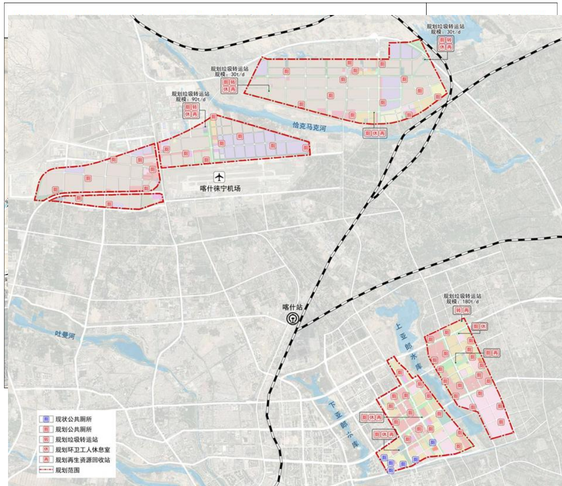
图2-3-19 伊尔克什坦口岸园区环卫设施工程规划图
