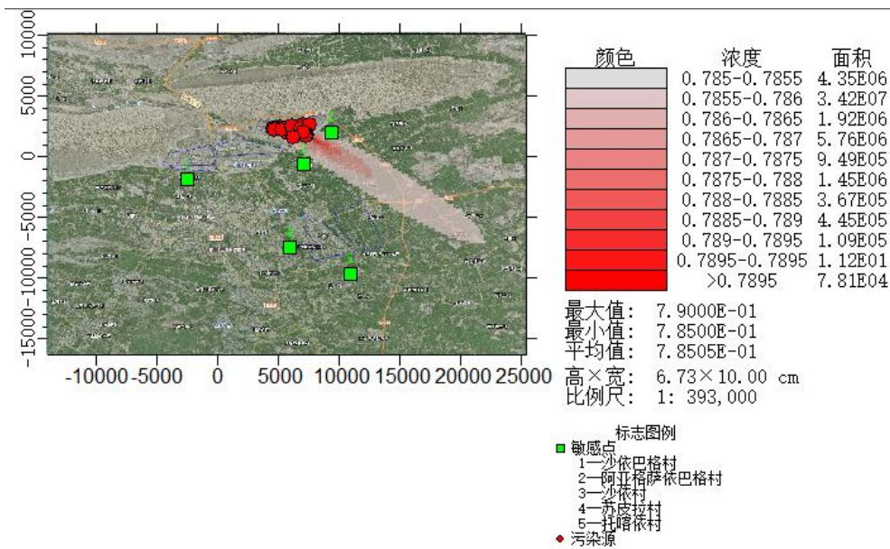
图5-2-10 非甲烷总烃小时值落地浓度叠加值网格图 (mg/m 3 )
