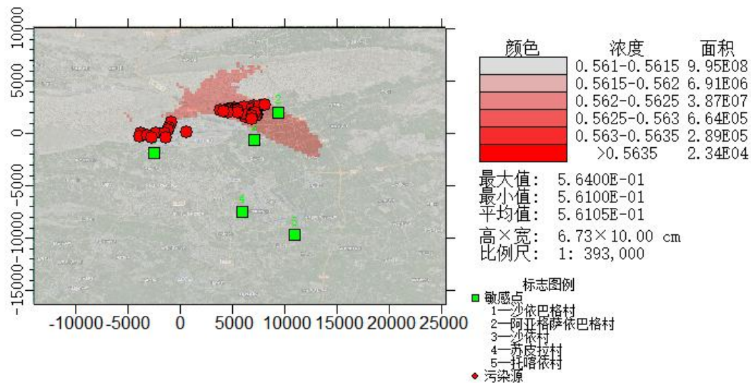
5-2-12 NO 2 年均落地浓度叠加值网格图 (mg/m 3 )
