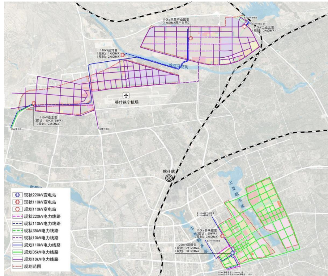
图 2-3-8 喀什经济开发区（主体园区）供电工程规划图
