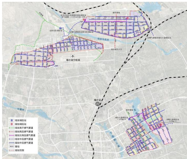
图2-3-14 喀什经济开发区（主体园区）燃气工程规划图
